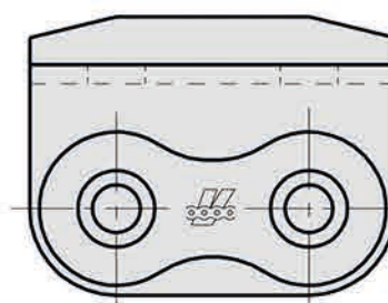
PROFIL "F1"
